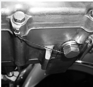
ワイヤーロック（緩み防止） ※ワイヤーは、ねじを締める方向へかけてください。
